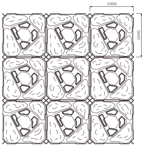
横断面図
