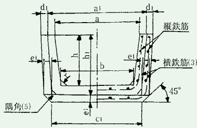
ソケット部断面
